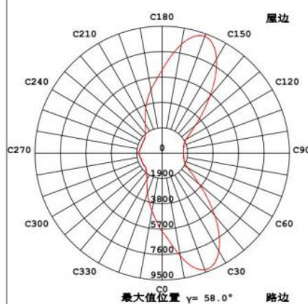
最大光强处圆锥面光强分布曲线
